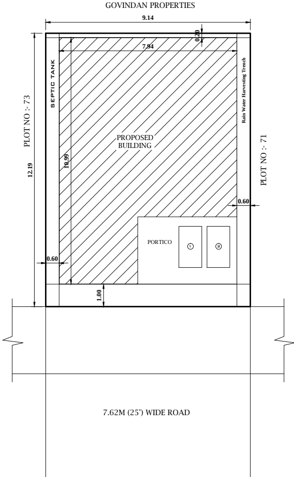
SITE PLAN 1:100
