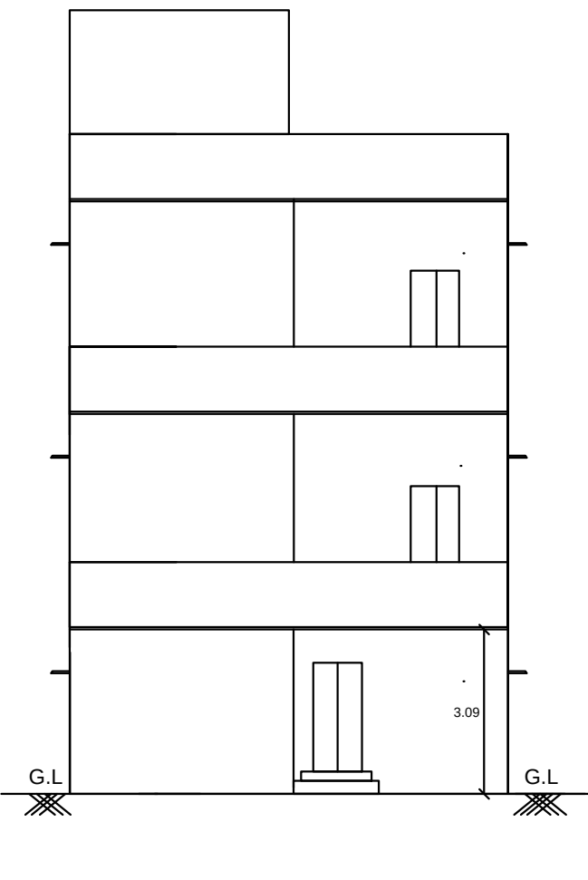
ELEVATION
