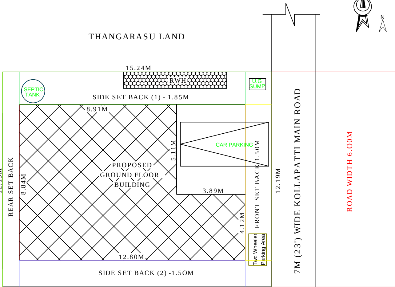
SITE PLAN :
