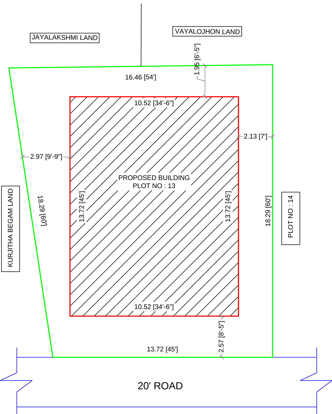
SITE PLAN ( 1:100)
