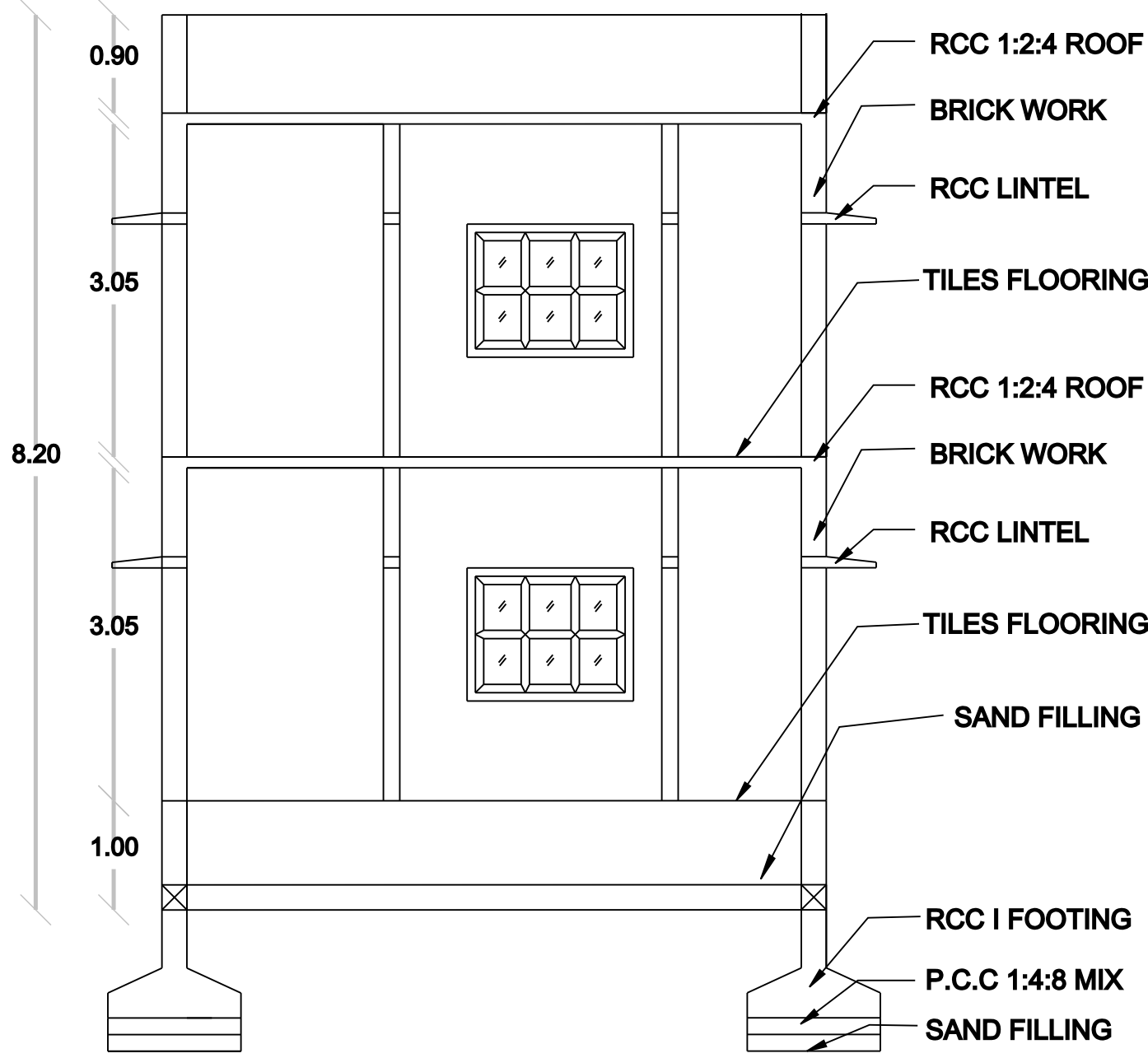
SECTION A-B
