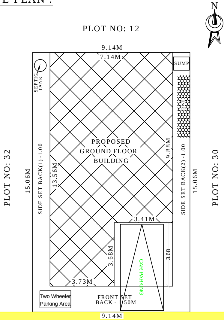
SITE PLAN :
