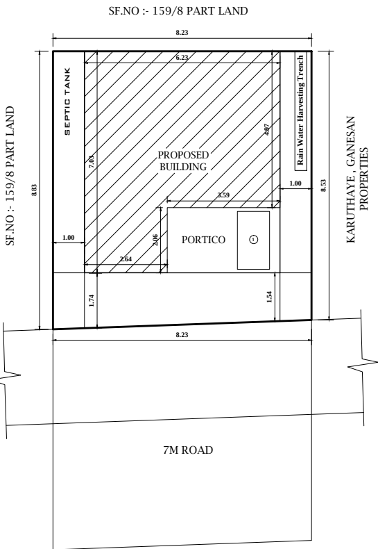
SITE PLAN 1:100
