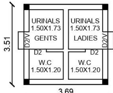
TOILET PLAN
