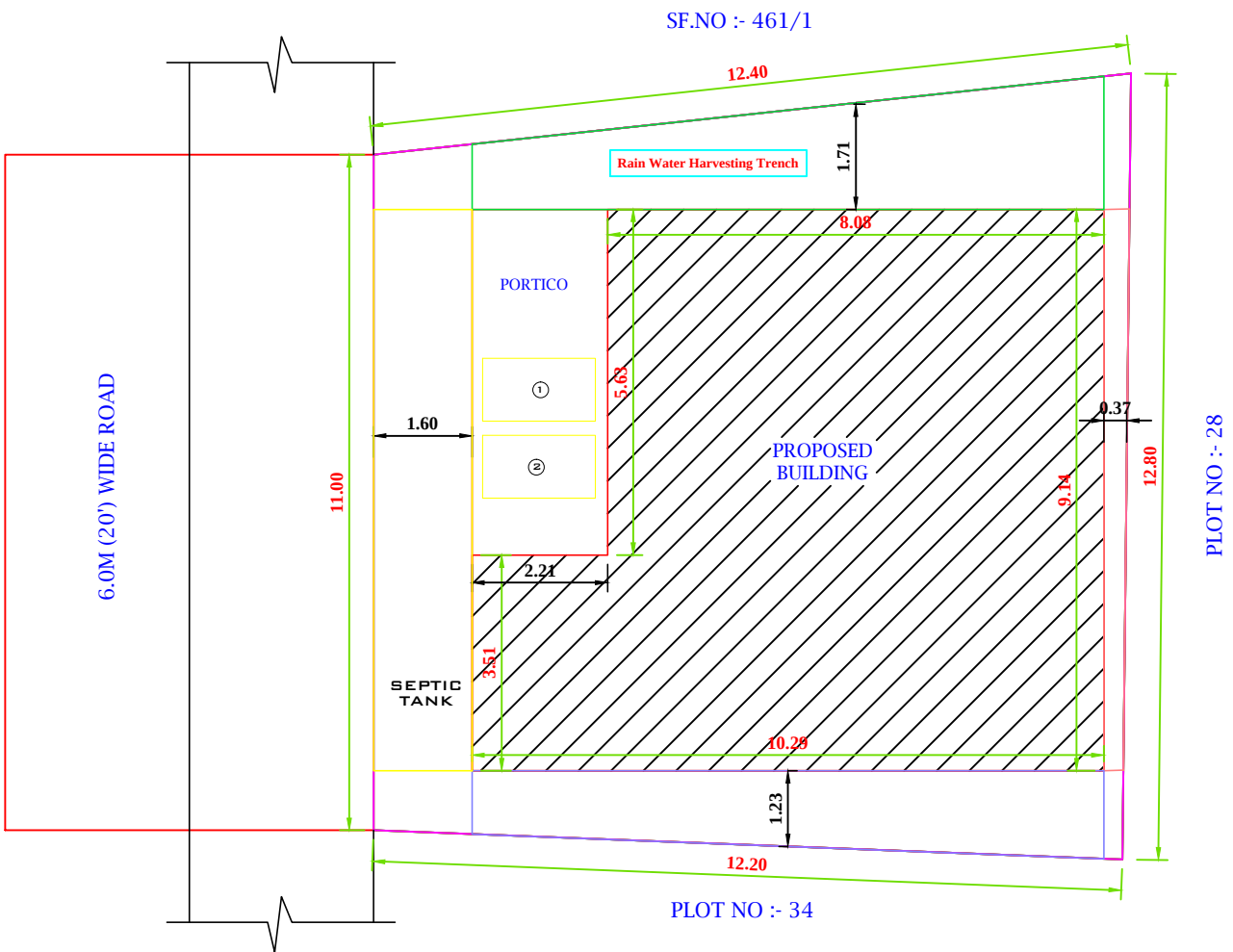
SITE PLAN 1:100
