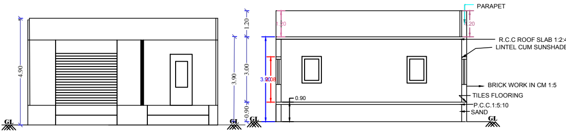
ELEVATION
