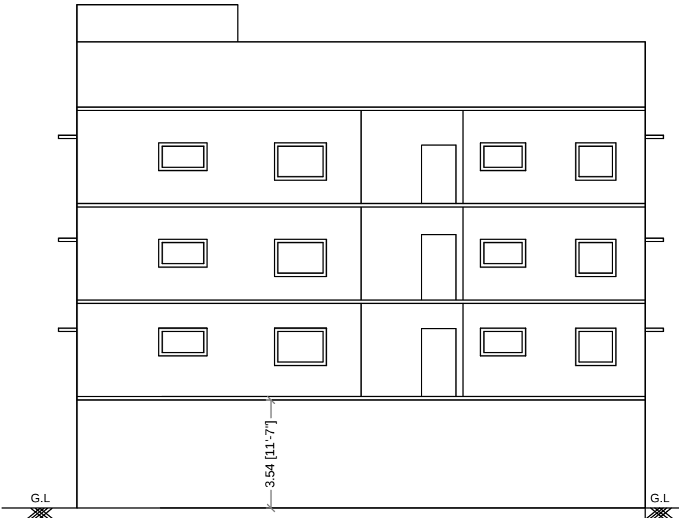
ELEVATION
