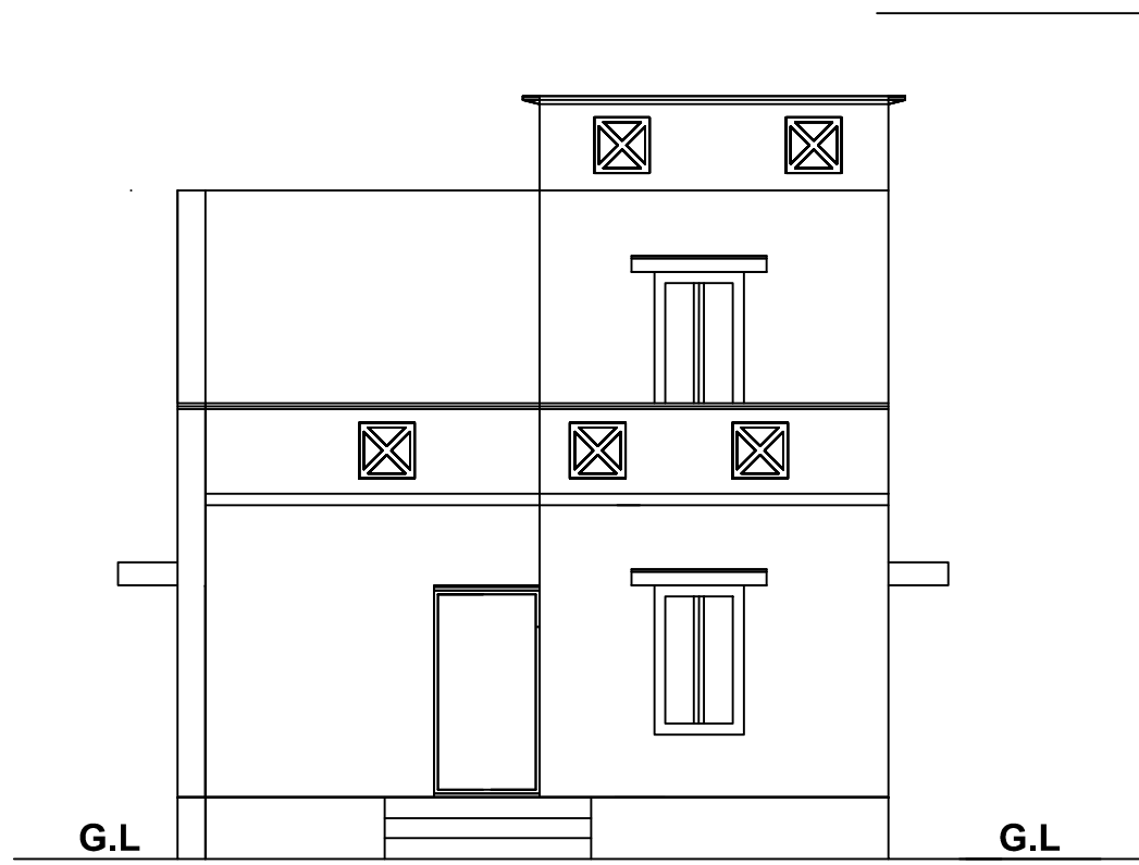
ELEVATION
