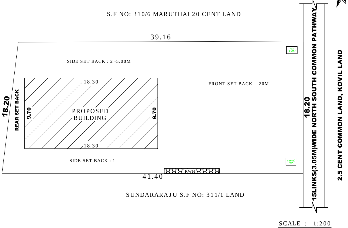
SITE PLAN :
