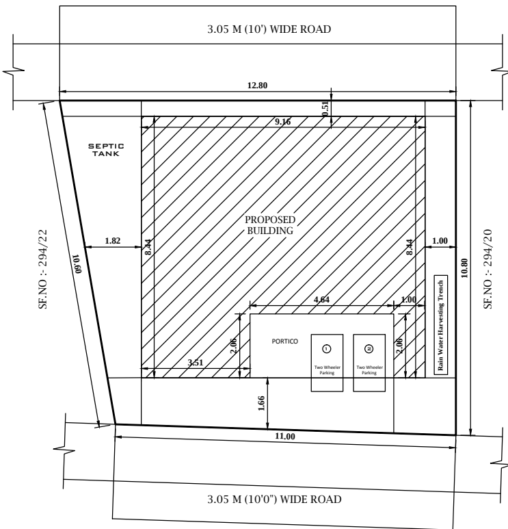
SITE PLAN 1:100
