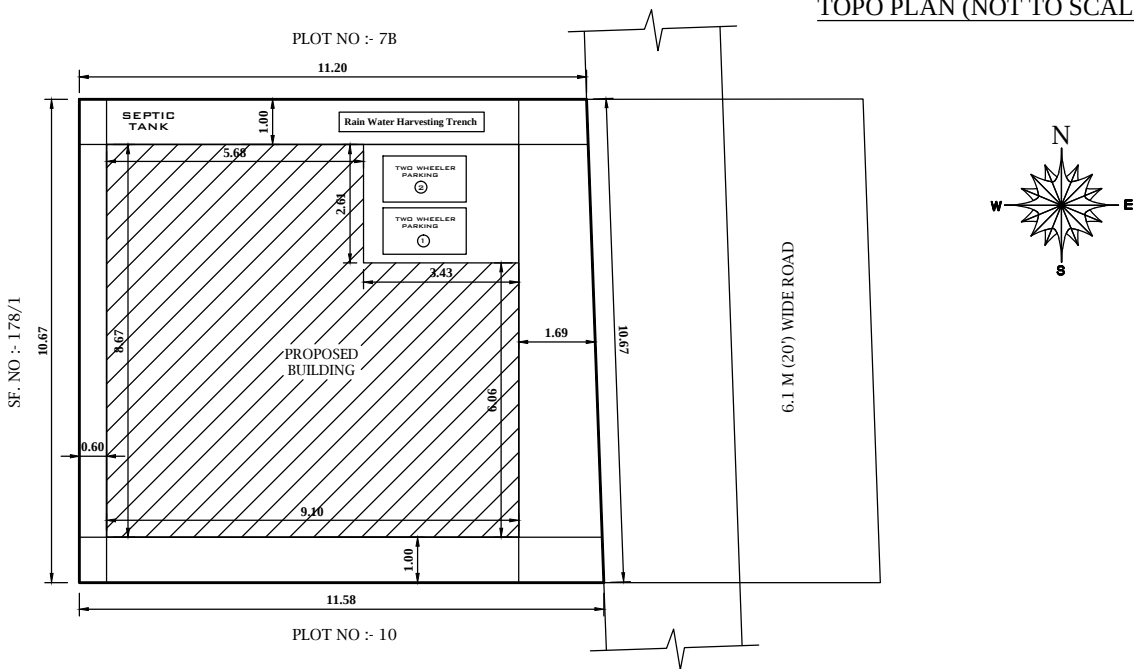
SITE PLAN 1:100
