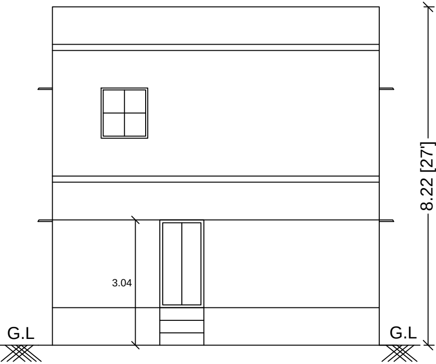
ELEVATION
