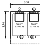
TOILET PLAN
