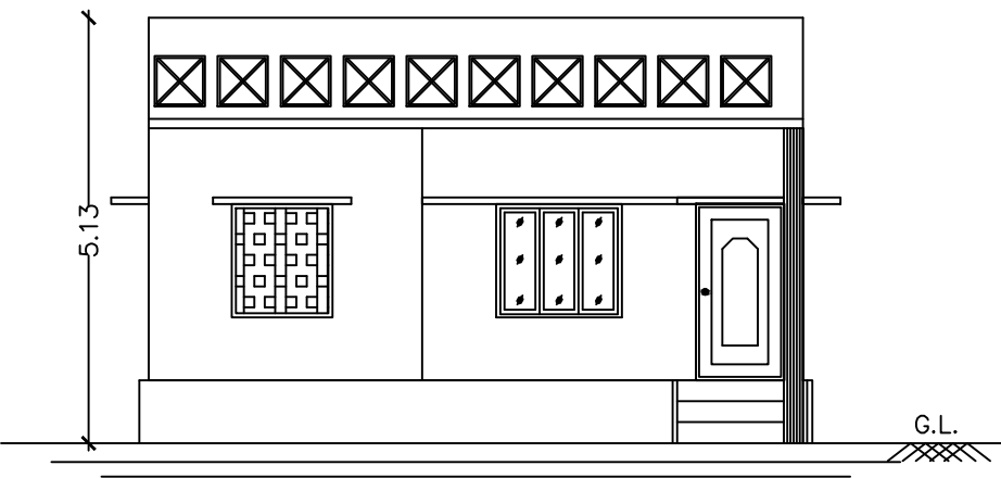
ELEVATION
