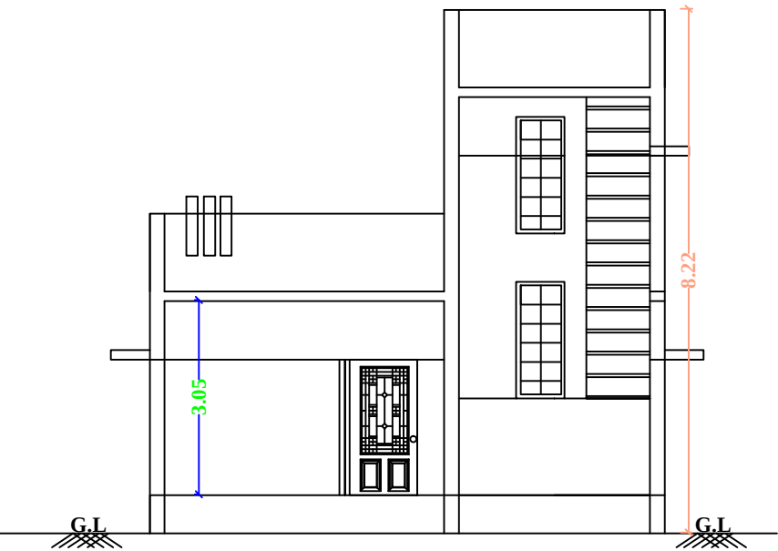
ELEVATION
