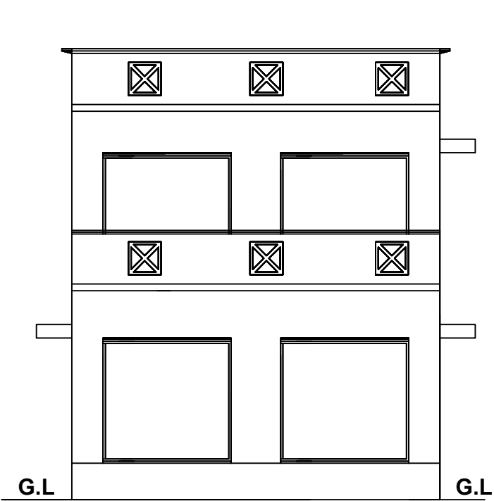
ELEVATION
