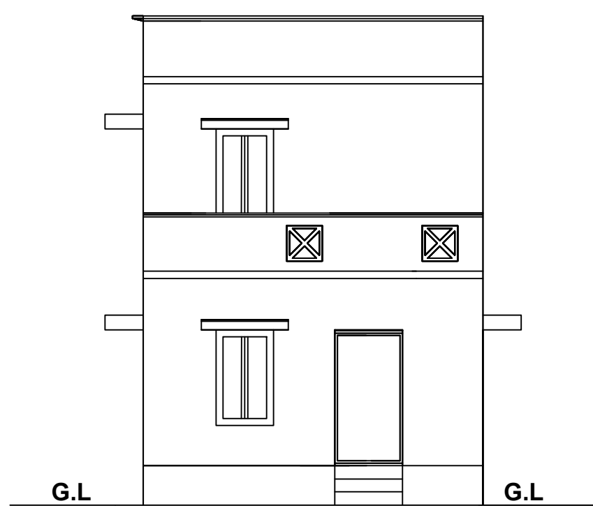
ELEVATION
