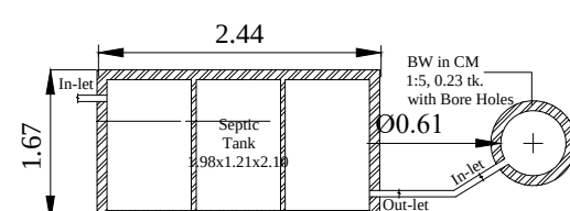
SOAK PIT
