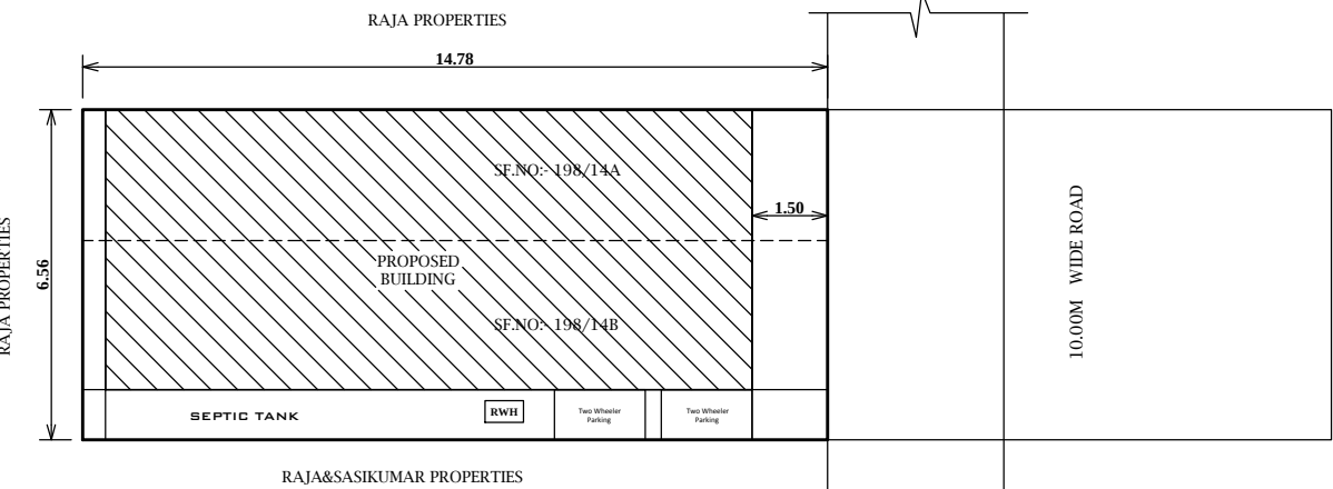
SITE PLAN 1:100
