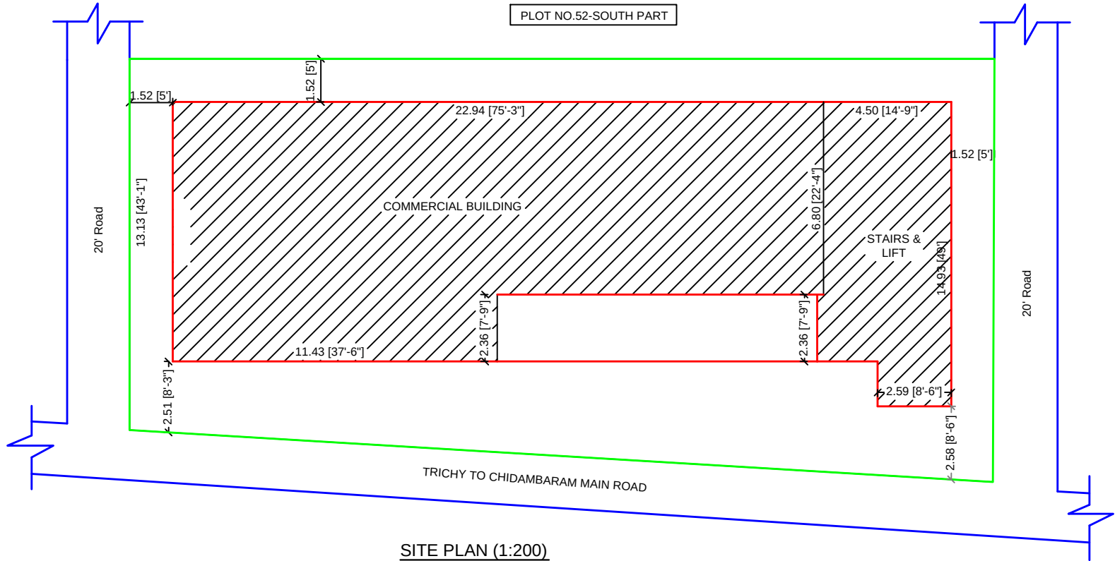
SITE PLAN (1:200)
