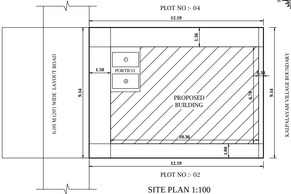
SITE PLAN 1:100
