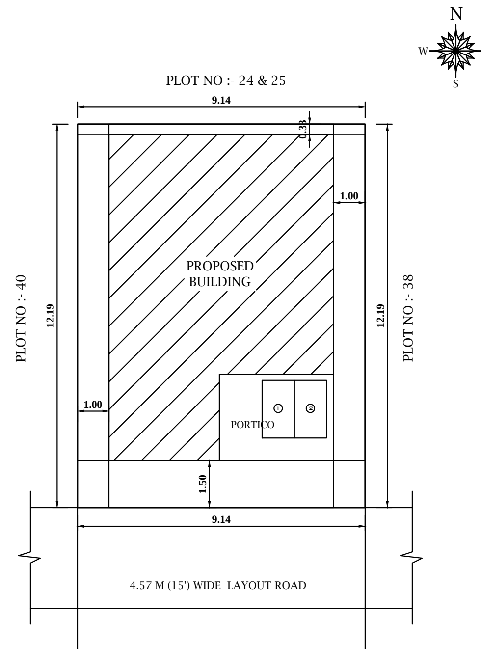
SITE PLAN 1:100
