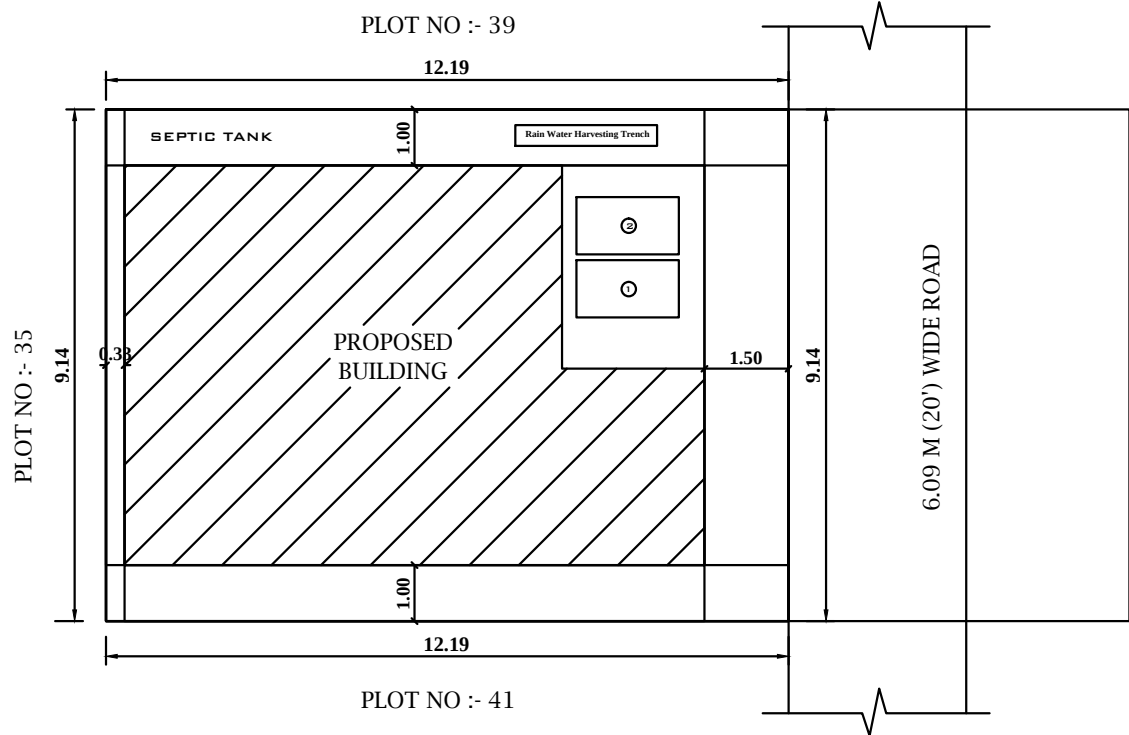
SITE PLAN 1:100
