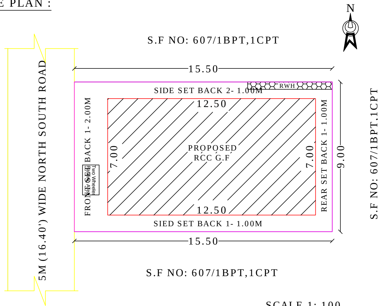
SITE PLAN :
