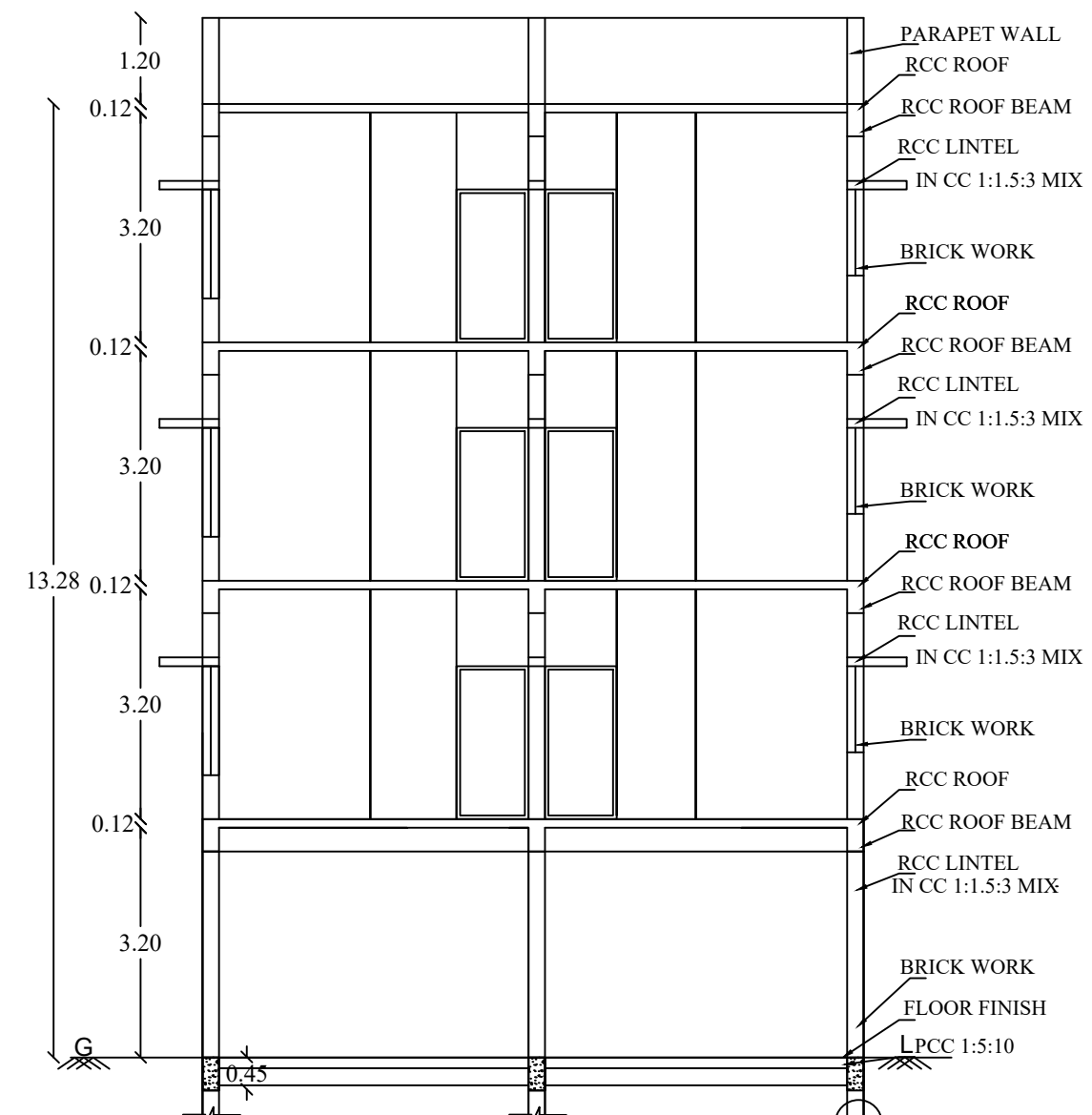
SECTION - AB
