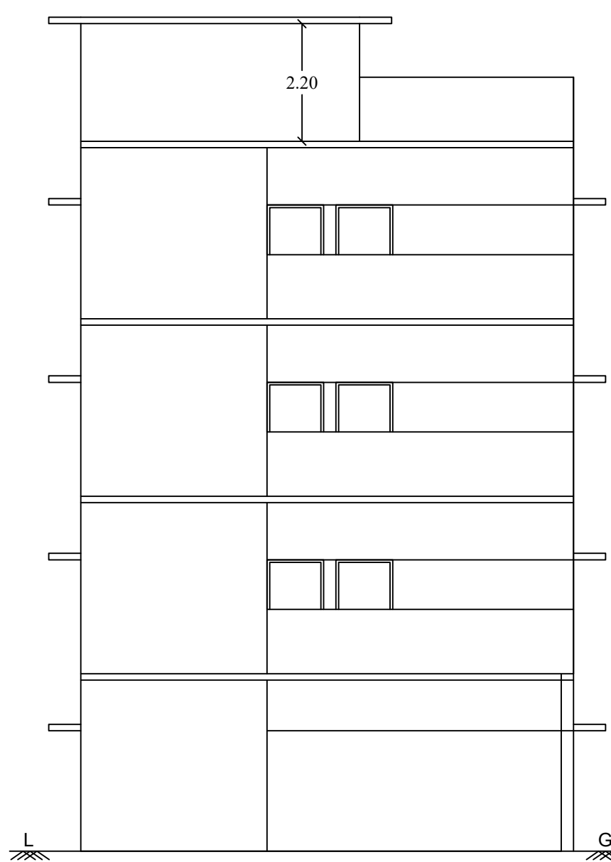
ELEVATION
