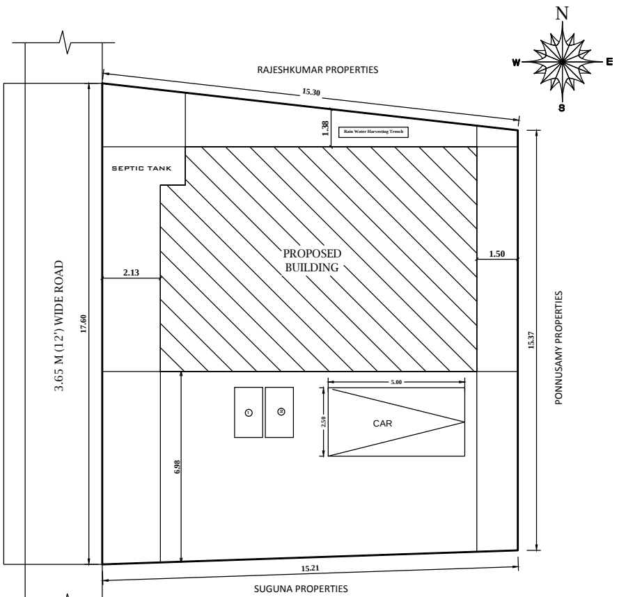
SITE PLAN 1:100
