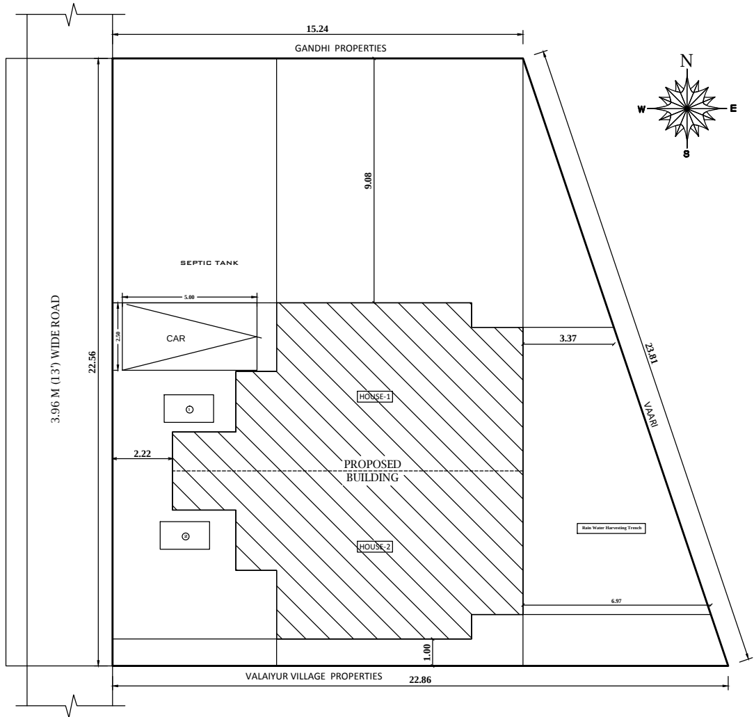
SITE PLAN 1:100
