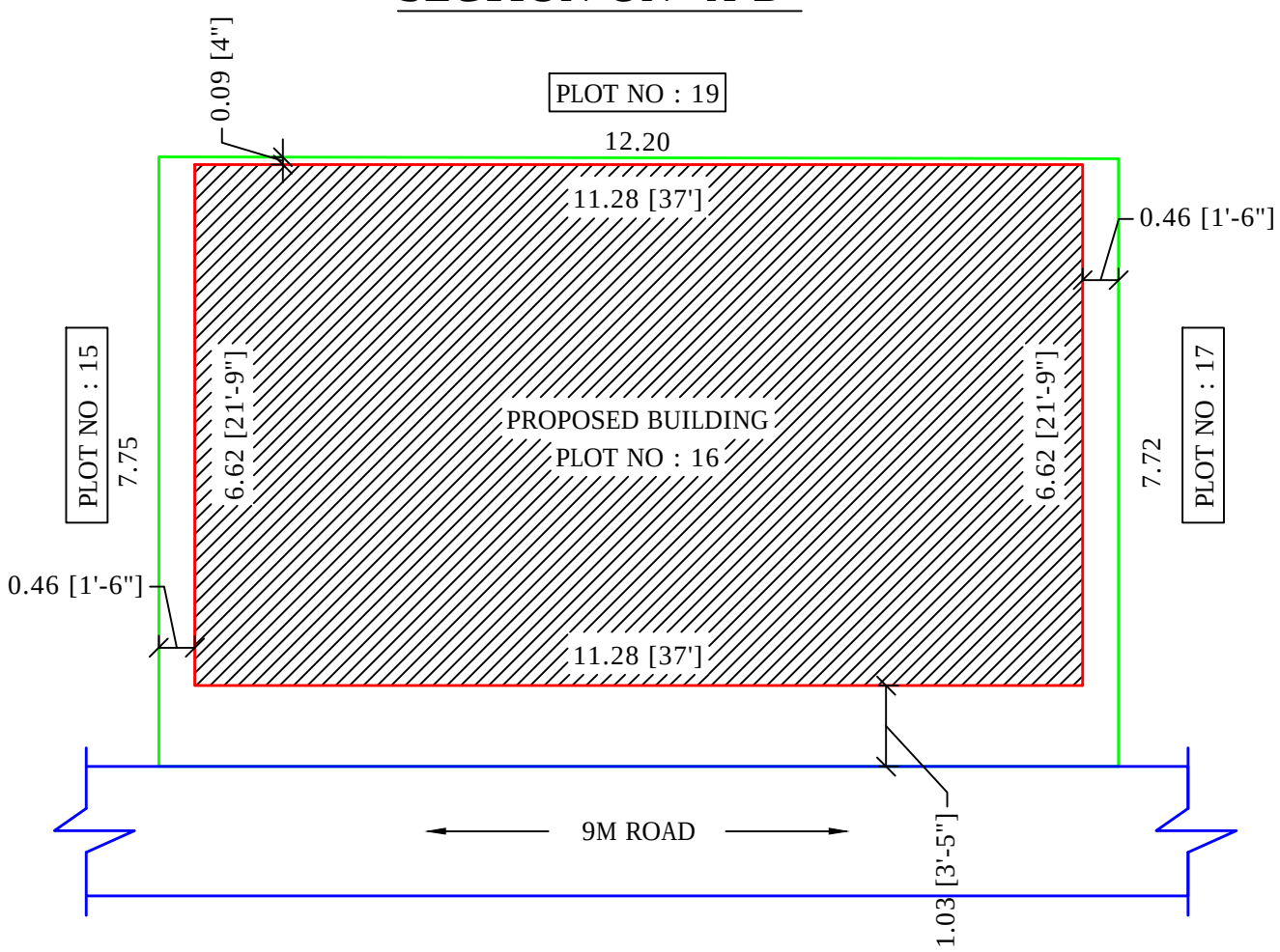
SITE PLAN ( 1:100 )
