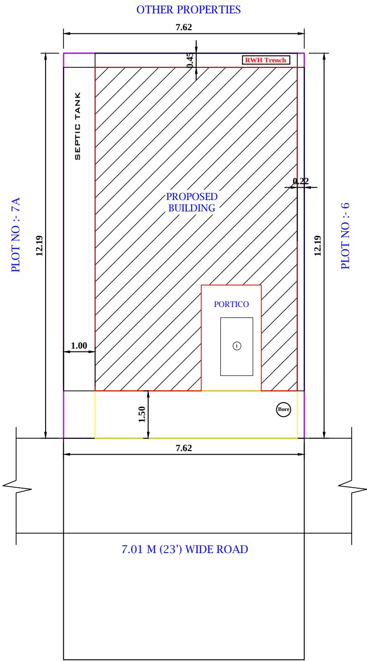
SITE PLAN 1:100
