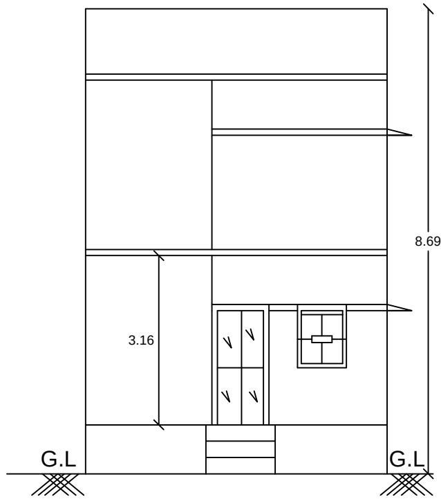
ELEVATION
