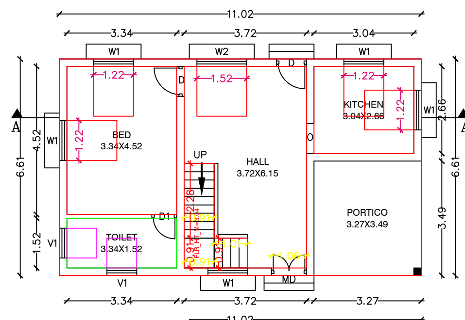
UND FLOOR PLAN
