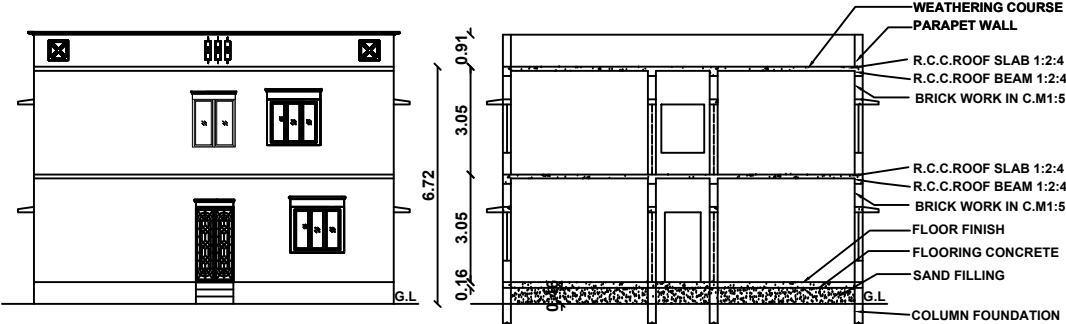
ELEVATION
