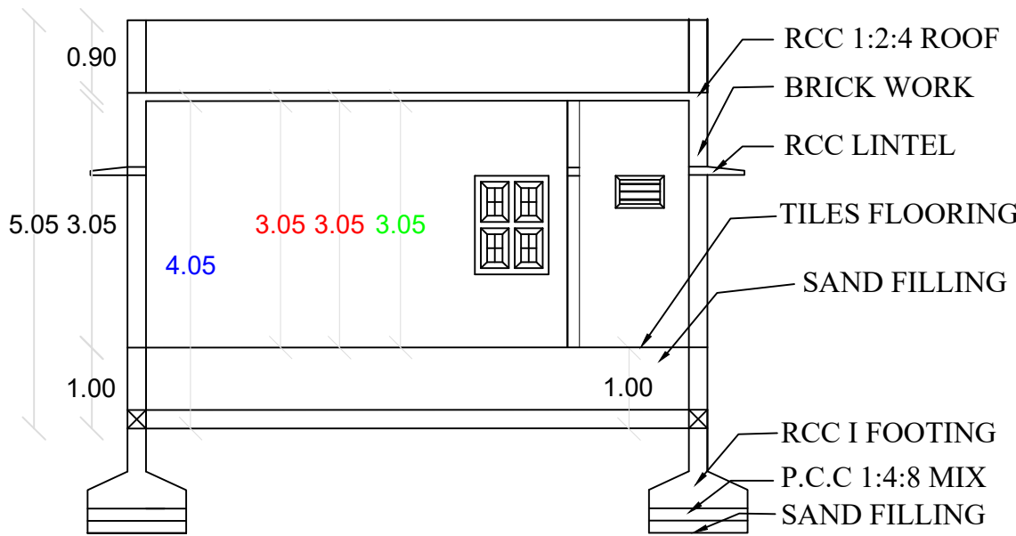
SECTION A-B
