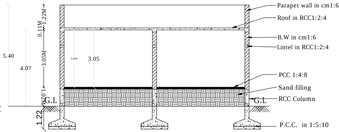
SECTION - AB
