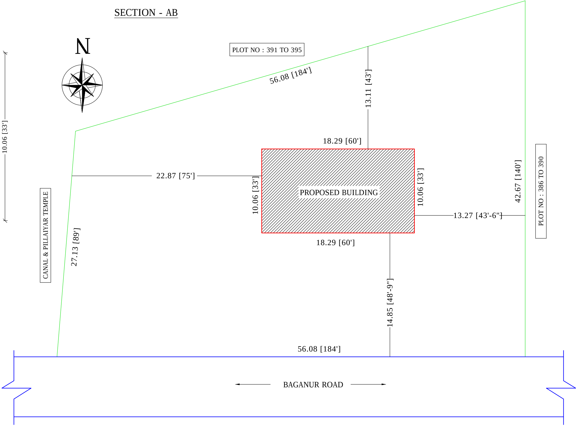
SITE PLAN ( 1:200 )
