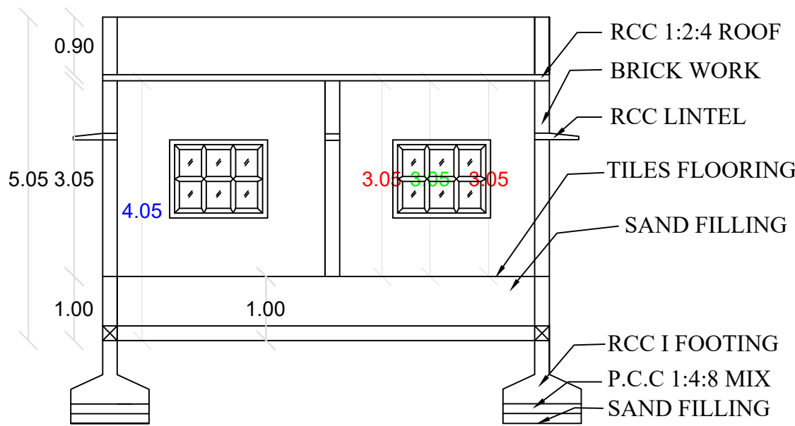
SECTION A-B
