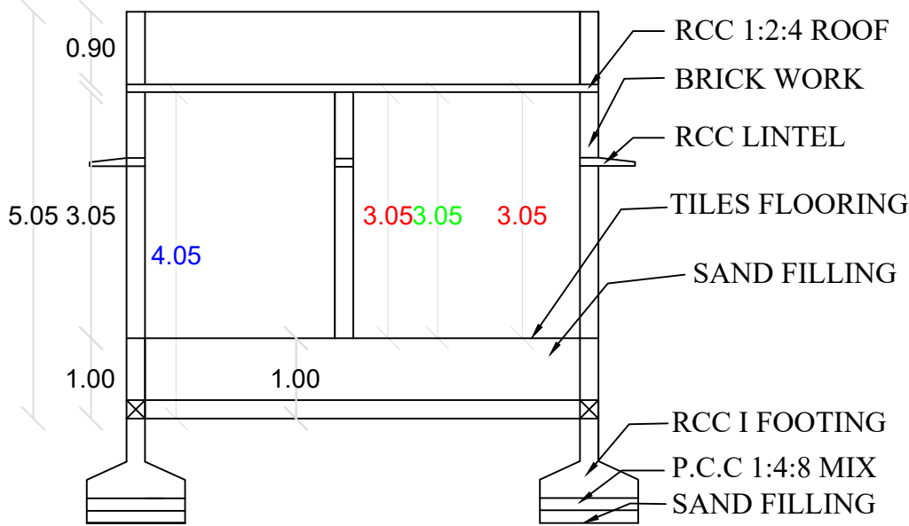
SECTION A-B
