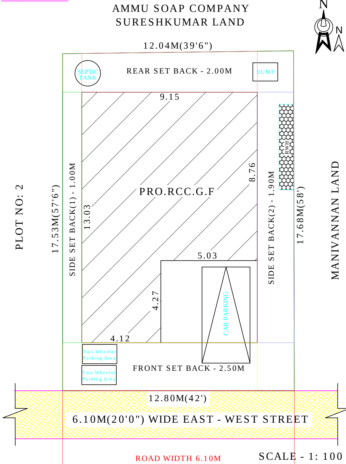
SITE PLAN:
