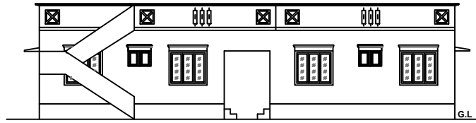
ELEVATION
