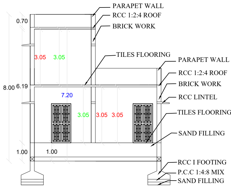
SECTION A-B
