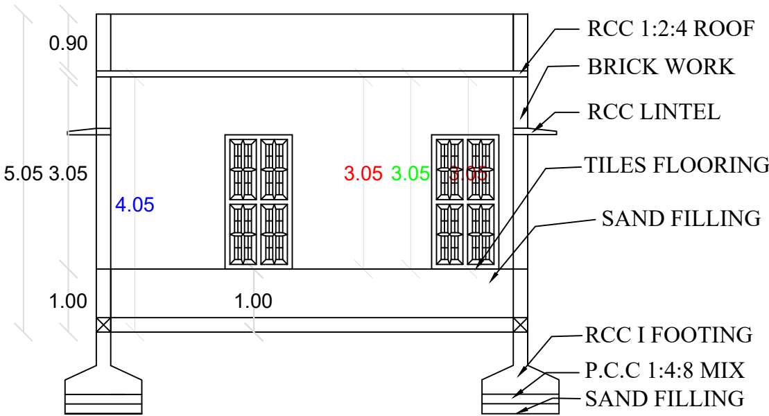
SECTION A-B
