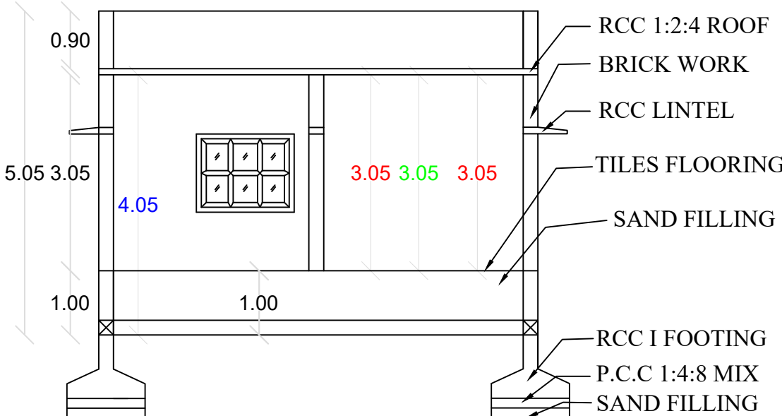
SECTION A-B
