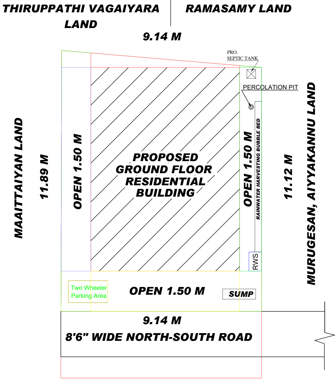
SITE PLAN (SCALE: 1:1)
