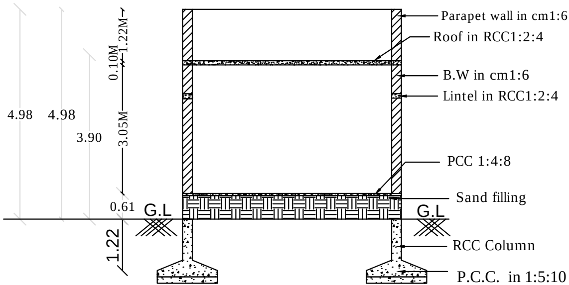
SECTION - AB
