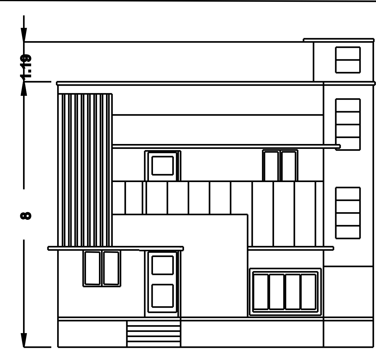
ELEVATION - A
