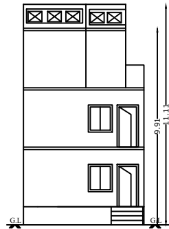
ELEVATION
