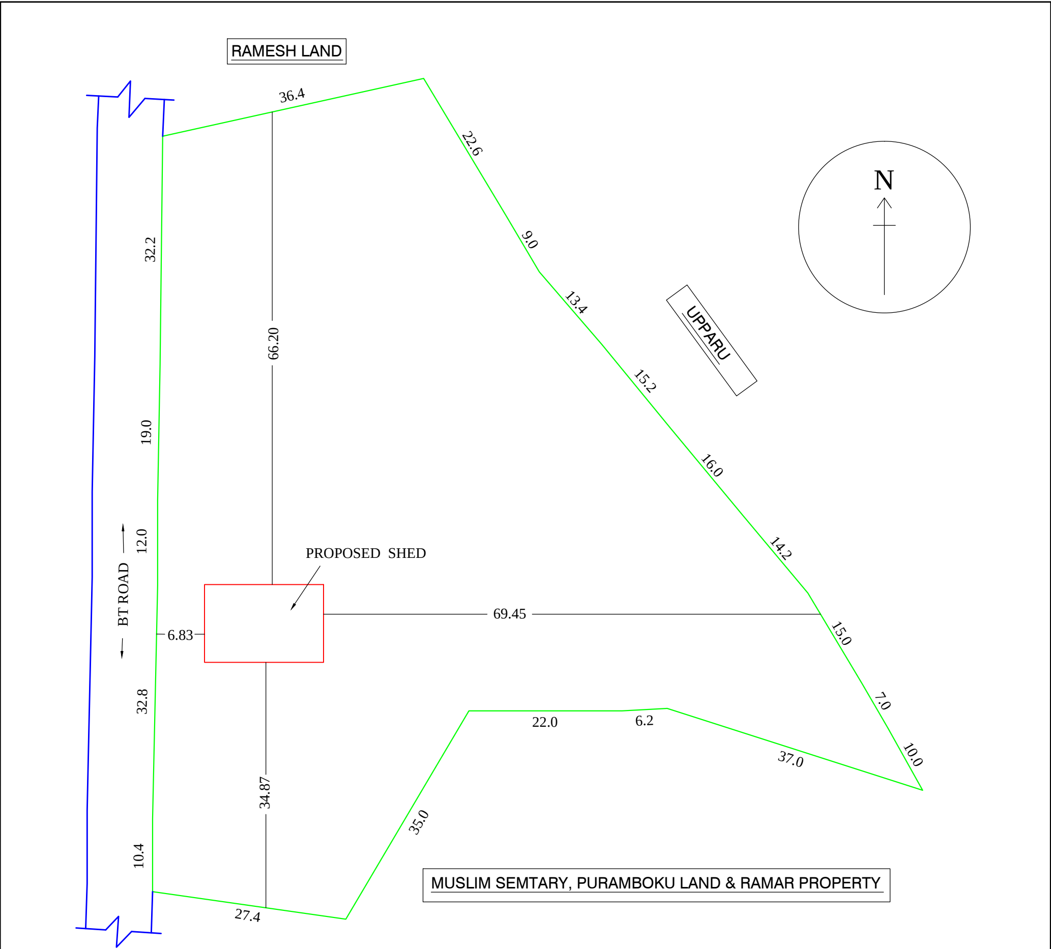
SITE PLAN ( 1: 400)
