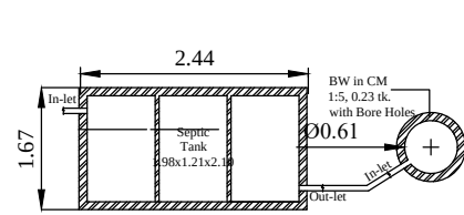
SOAK PIT
