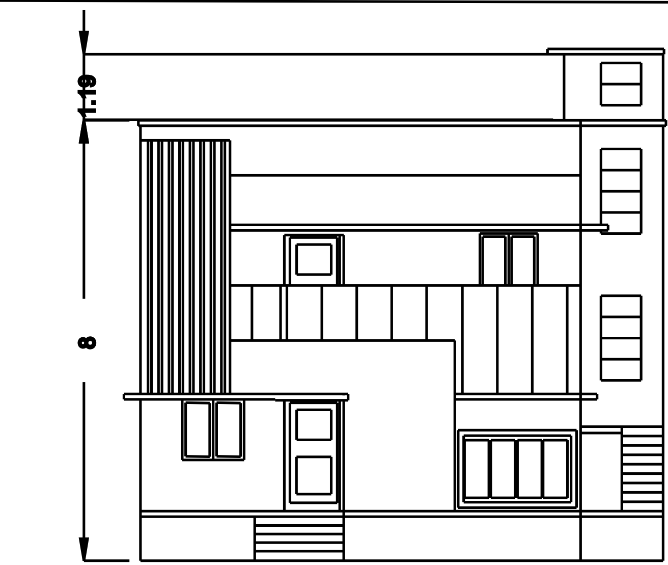
ELEVATION - A
